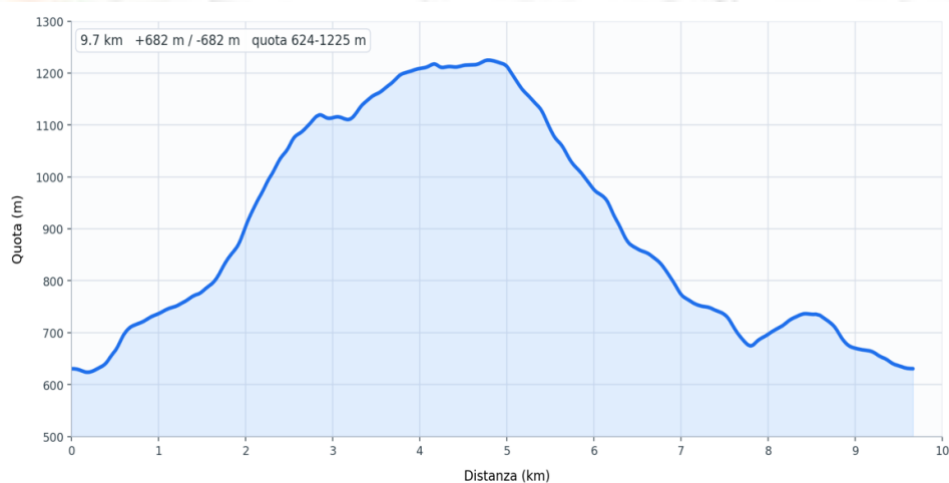
Profilo altimetrico
